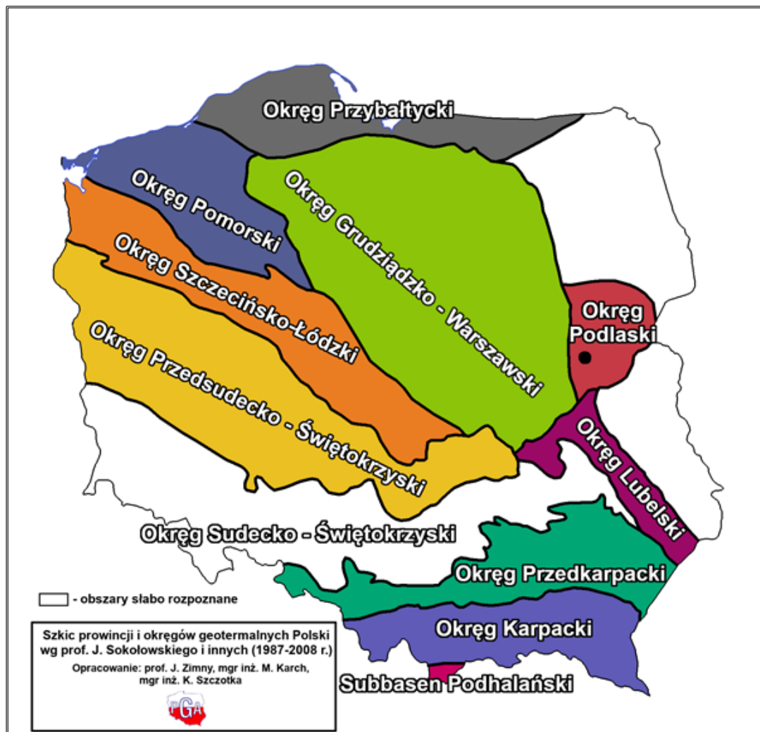
Rysunek 6. Położenie miasta Siedlce na tle okęgów geotermalnych Polski.
