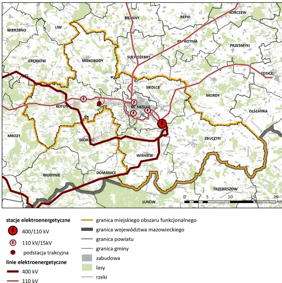
Rysunek 30 Sieć elektroenergetyczna
